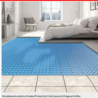
Riscaldamento elettrico Prodeso® Heat Grip 5 Stick System di Progress Profiles
