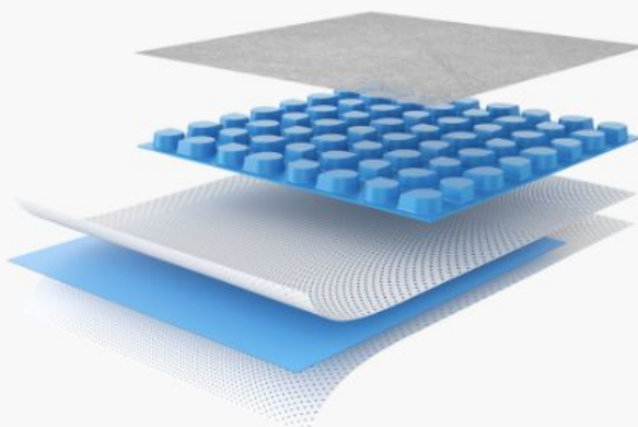
I cinque strati della membrana Prodeso® Drain 8 System di Progress Profiles
