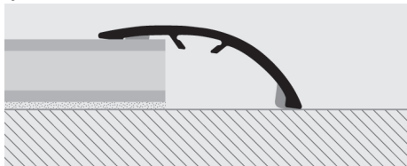
ALUMINIO REVESTIDO 80 acabados madera (49 solo bajo pedido) con ADHESIVO - ancho 40 mm - Unidades de 2,7 M de largo - Paq. de 40 UDS - 108 M
