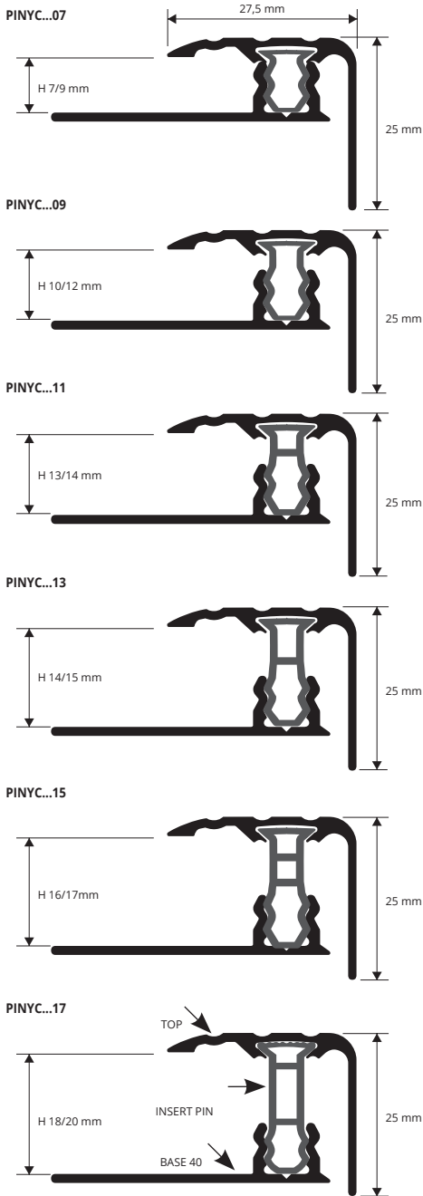
TOP ALU. + INSERT PIN + BASE 40 ALU. COUPÉE/PERFORÉE (6 finitions alu. anod. 3 sur demande) thermo packed long. b. 2,7 ML - cond. 20 Pces - 54 ML (H 14 - H 16 - H 18mm - 40,5 ML)
