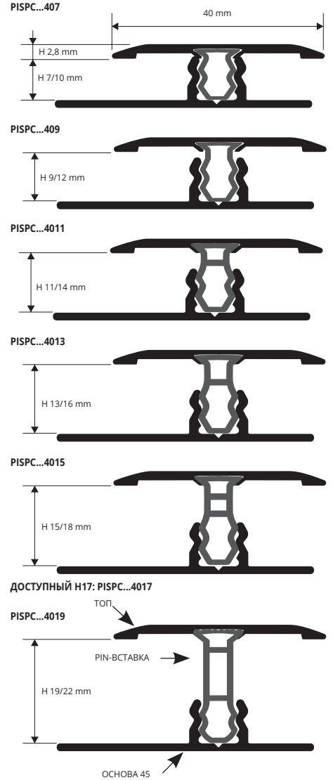
ДОСТУПНЫЙ Н17: PISPC...4017 PISPC...4019 ТОП PIN-ВСТАВКА ОСНОВА 45 H 19/22 mm
