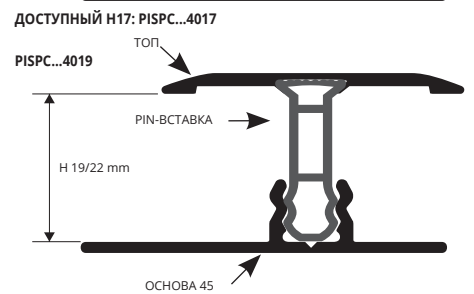
ДОСТУПНЫЙ Н17: PISPC...4017 PISPC...4019 ТОП PIN-ВСТАВКА ОСНОВА 45 H 19/22 mm
