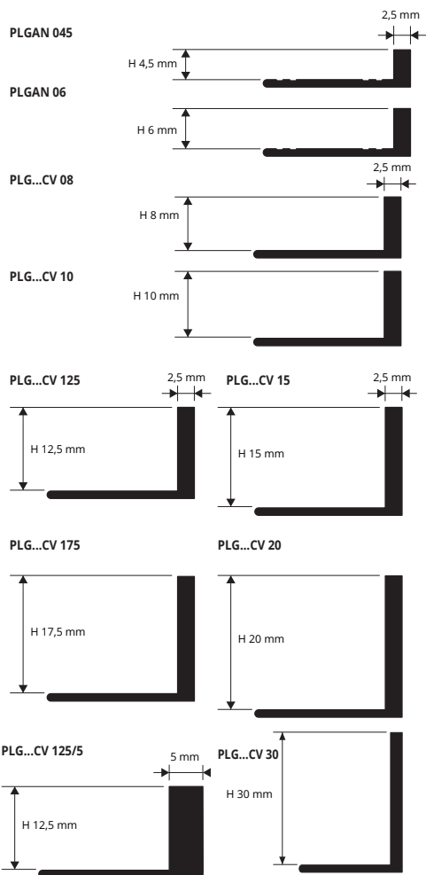
OTTONE NATURALE thermo packed 10 PZ lung. barre 2,7 ml - conf. 20 PZ - 54 ml
